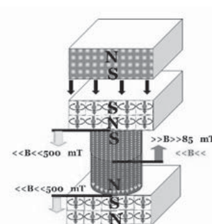
<<B<< Antifusha magnetike <<B<< Fusha magnetike (N-S) >>B>> Fusha magnetike qendër të magnetit
